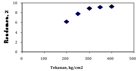
Gambar 3. Grafik hubungan Tekanan dengan Rendemen
