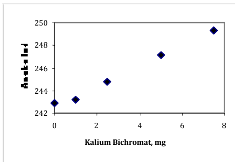
Gambar 5. Grafik hubungan Kadar Kalium Bichromat terhadap Angka Iod.
