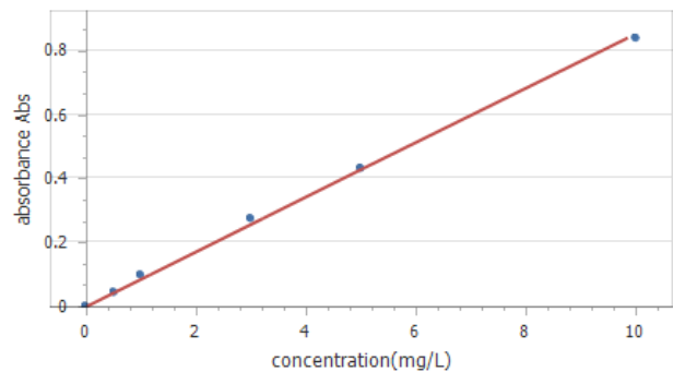
Gambar 7. Grafik Kurva Kalibrasi Ag
