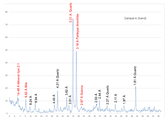
Gambar 4. Grafik Hasil Tes XRD Sampel A (Pasir)
