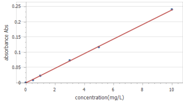
Gambar 6. Grafik Kurva Kalibrasi Au
