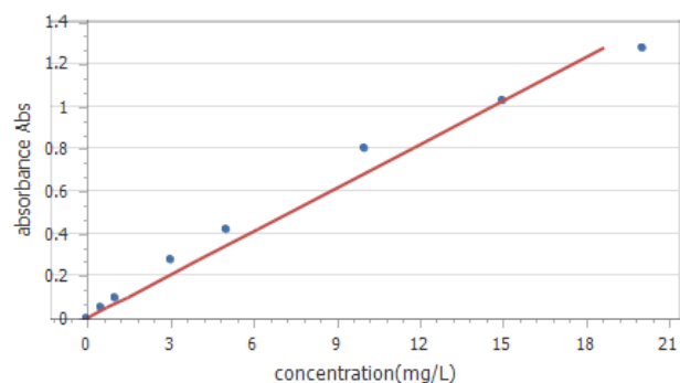
Gambar 8. Grafik Kurva Kalibrasi Cu
