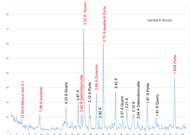
Gambar 5. Grafik Hasil Tes XRD Sampel B (Batuan)
