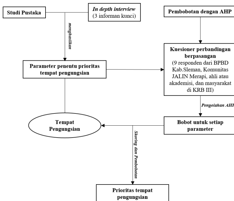
Gambar 2. Tahapan Penelitian
