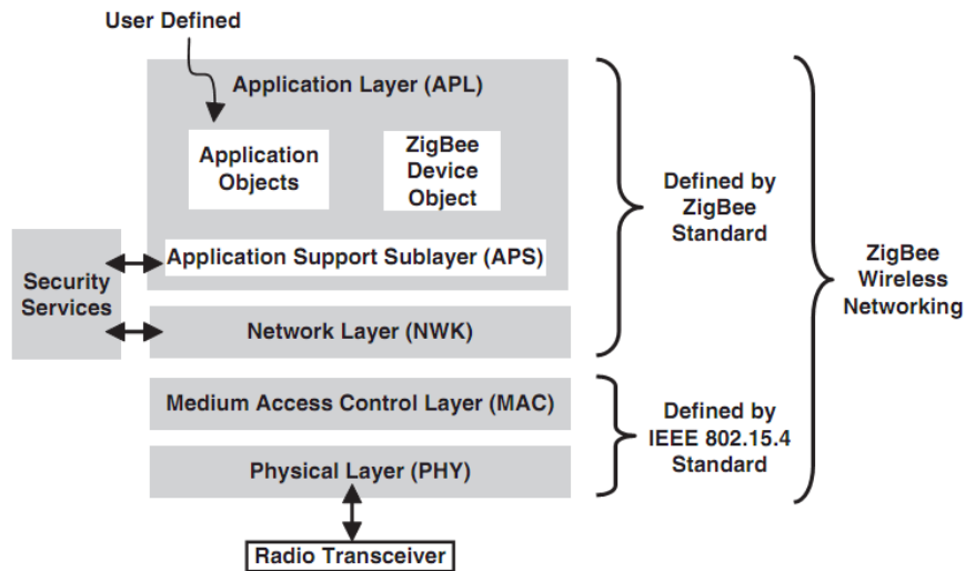
Gambar 1. Hubungan antara ZigBee dan IEEE 802.15.4
