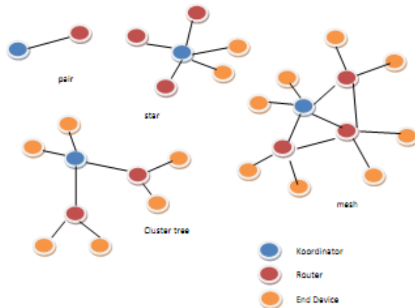
Gambar 2. Topologi jaringan ZigBee
