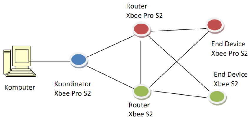
Gambar 3. Konfigurasi jaringan.
