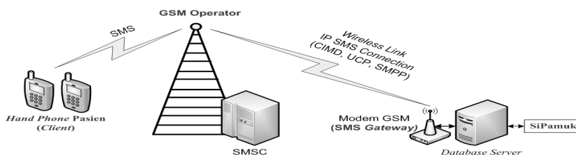
Gambar 2. Arsitektur SiPamuk
