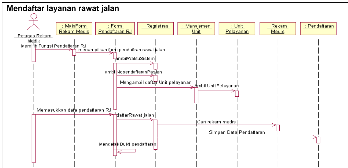
Gambar 8. Design Basic Flow Mendaftar Pasien Rawat Jalan (Sequence Diagram)
